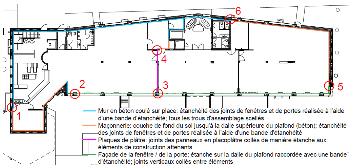
Illustration 5 : Plan avec inscription des mesures relatives à l'étanchéité à l'air. Source : plans mis à disposition par Flumroc SA.
