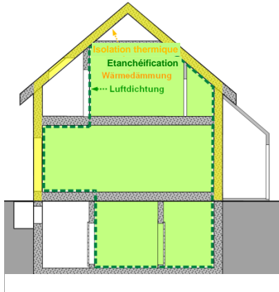
Illustration 11 : Pour les maisons individuelles plus anciennes, il convient de définir où passe le périmètre d'étanchéité.
