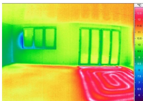
Illustration 22 : Différence de température à travers l'enveloppe du bâtiment : environ 8 K, dépression : 50 Pa, depuis environ 10 min. Attention : la fenêtre de gauche est étanche ! La raison de la tache bleue et froide sur la gauche : la fenêtre était en imposte avant la mesure (Source :Ingenieurbüro Bauchecheck-Tanner)
