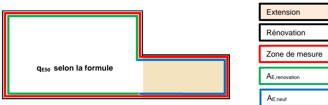
Illustration 17 : « Mélange de mesures » de la rénovation et de l'extension en tant qu'ébauche du système. P.ex. annexe ouverte (p.ex. maison individuelle avec extension de pièce)
