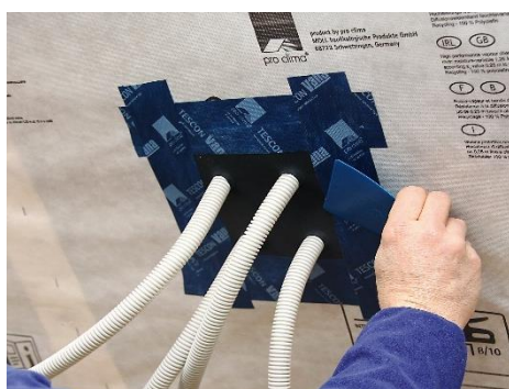
Illustration 10 : Manchette appropriée pour gaines multiples (source : image gauche : pro clima Suisse GmbH, image droite : Kel-DPU)
