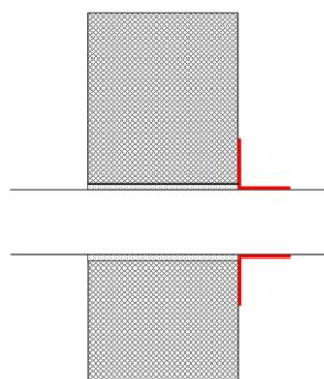
Illustration 7 : Exemple typique de pénétration autour d'un tuyau
