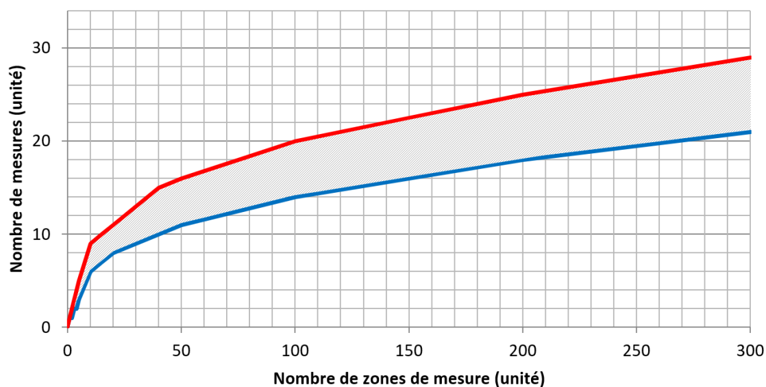
Illustration 13 : Graphique illustrant la fourchette du nombre de mesures devant être réalisées
