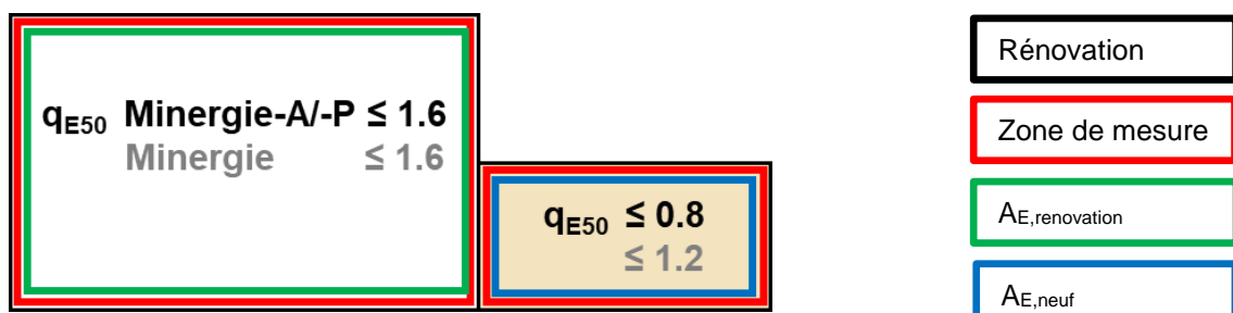
Illustration 15 : Mesures séparées de la rénovation et de l'extension en tant qu'ébauche du système. P.ex. annexe indépendante
