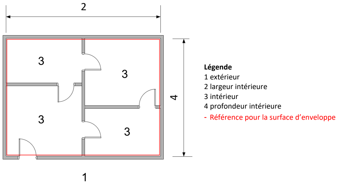
Illustration 18 : Plan avec représentation des dimensions intérieures globales (source : SN EN ISO 9972 ; 2015)
