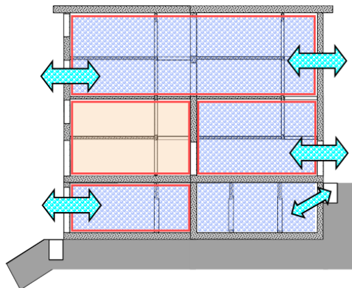
Illustration 20 : Mesure d'une unité d'utilisation (logement) dans un bâtiment (maison collective). Les fenêtres des logements adjacents, de la cage d'escalier et des locaux annexes non chauffés doivent être ouvertes.
