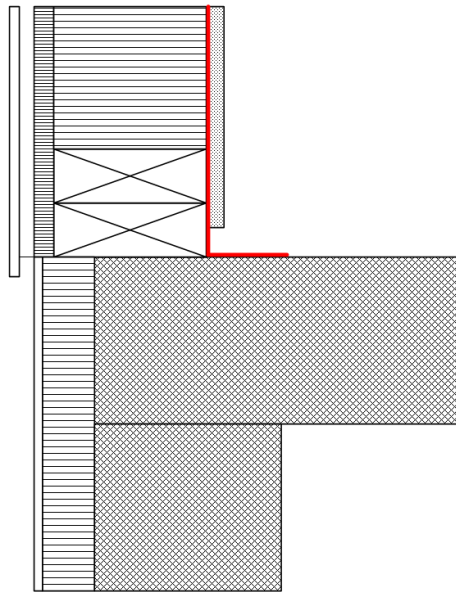
Illustration 6 : Exemple typique de raccords sol - murs extérieurs au niveau des éléments de construction
