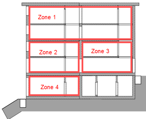
Illustration 12 : Immeuble collectif avec quatre unités d'utilisation. Dans les immeubles collectifs, chaque unité d'utilisation (logement, espace commun, etc.) doit être étanche à l'air par rapport aux autres unités d'utilisation. Cette indication s'applique aussi aux cages d'escalier, qui sont rarement mesurées en tant que zone séparée.
