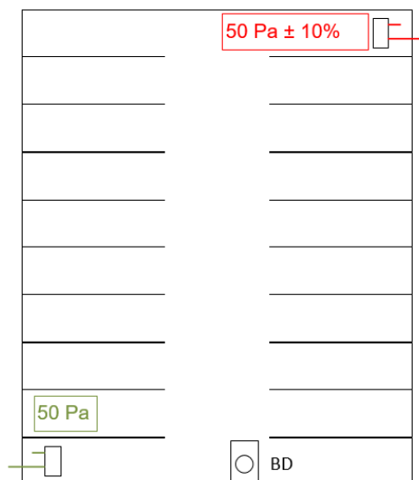
Illustration 25 : Graphique du contrôle de la différence de pression entre l'intérieur et l'extérieur dans les zones critiques
