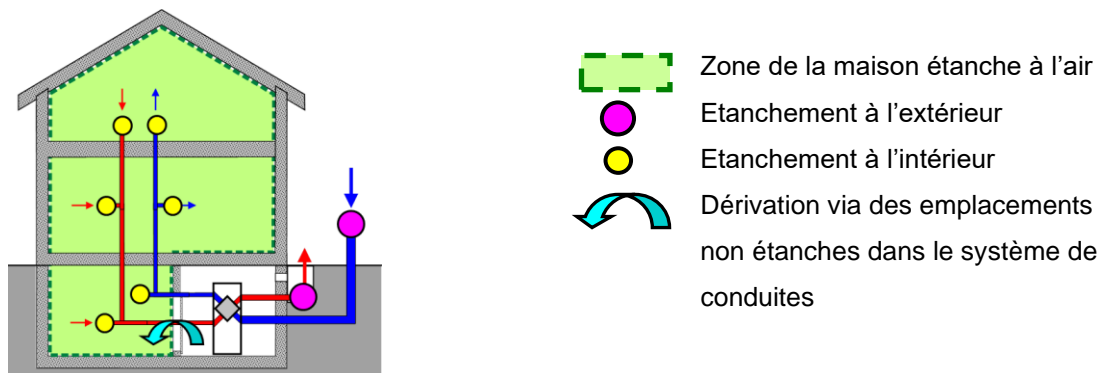
Illustration 23 : Étanchements provisoires possibles pour les installations de ventilation
