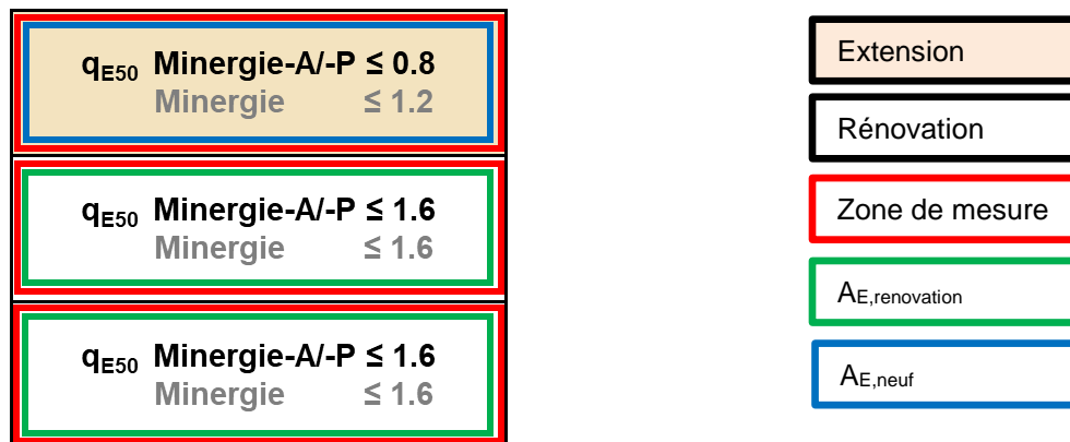
Illustration 14 : Mesures séparées de la rénovation et de l'extension en tant qu'ébauche du système. P.ex. surélévation indépendante
