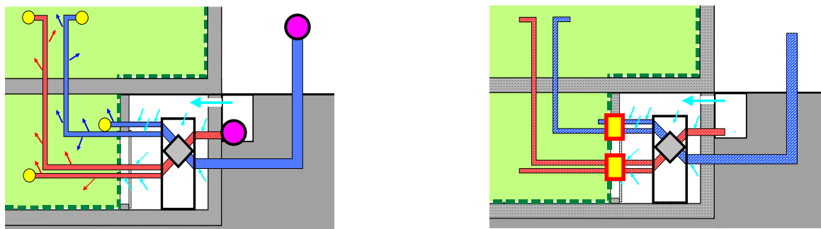
Illustration 24 : À gauche : des dérivations d'air se produisent à travers tous les raccords non étanches des canaux de ventilation.
