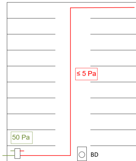
Illustration 26 : Graphique du contrôle de la différence de pression à l'intérieur du bâtiment
