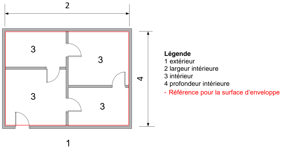
Illustration 18 : Plan avec représentation des dimensions intérieures globales (source : SN EN ISO 9972 ; 2015)
