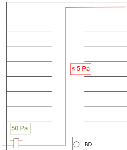
Illustration 26 : Graphique du contrôle de la différence de pression à l'intérieur du bâtiment ; Exemple de différence de pression dans un bâtiment de 50 Pa à l'endroit où est installé le dispositif de mesure
