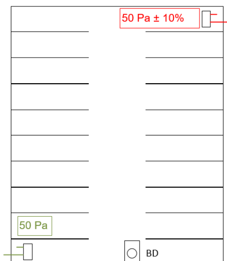
Illustration 25 : Graphique du contrôle de la différence de pression entre l'intérieur et l'extérieur dans les zones critiques ; Exemple de différence de pression dans un bâtiment de 50 Pa à l'endroit où est installé le dispositif de mesure
