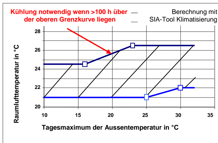
Abbildung 12: Nachweis für Notwendigkeit einer Kühlung gemäss SIA 382/1
